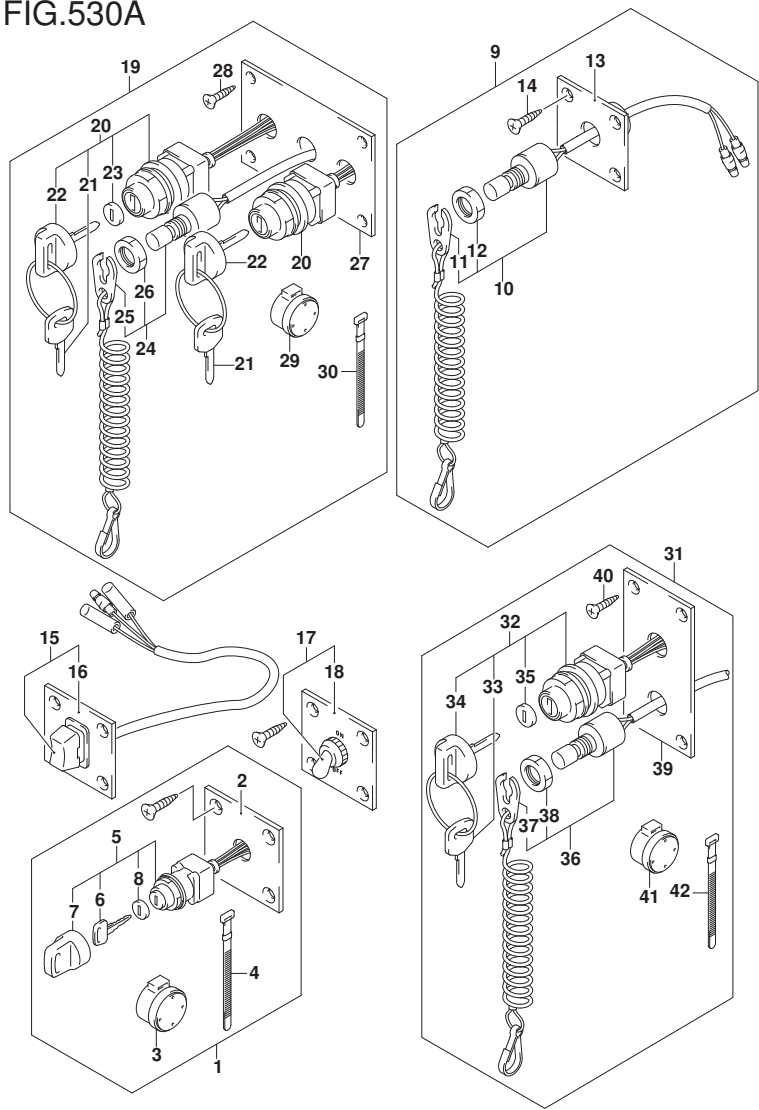
FIG.530A (1-H-6) OPT:SWITCH
